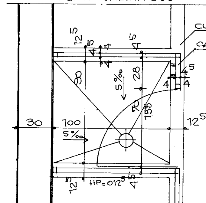
● SECTIUNE TRANSVERSALA ● PLAN CABINA DUS
