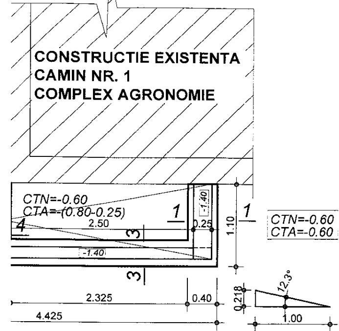
Detaliu - ancorare a barelor in centuri la intersectii
