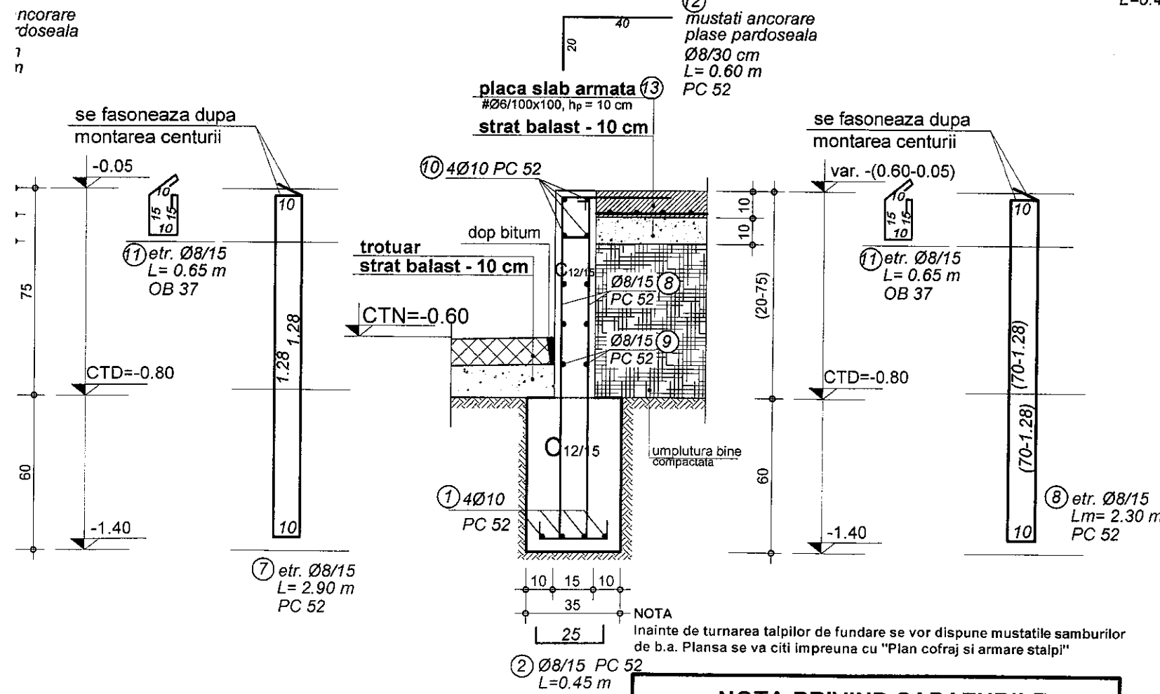
Detaliu rampa 3 - 3 SCARA 1:20
