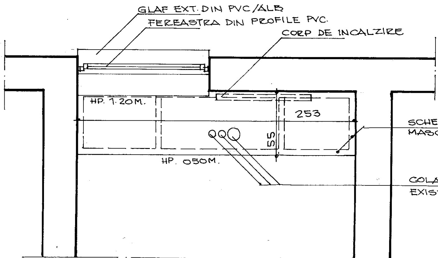
VEDERE ORIZONTALA sc.1:20
