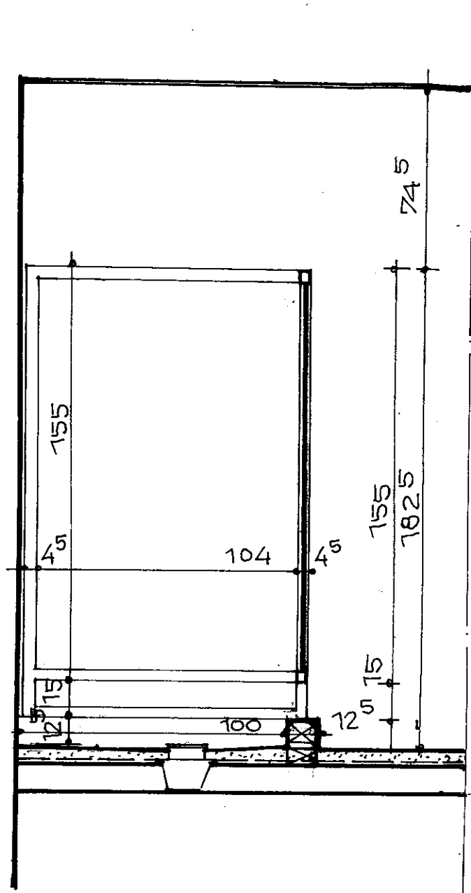
● SECTIUNE TRANSVERSALA ● PLAN CABINA DUS
