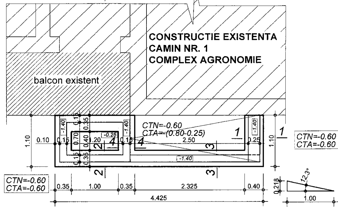
Detaliu rampa 2 - 2 SCARA 1:20
