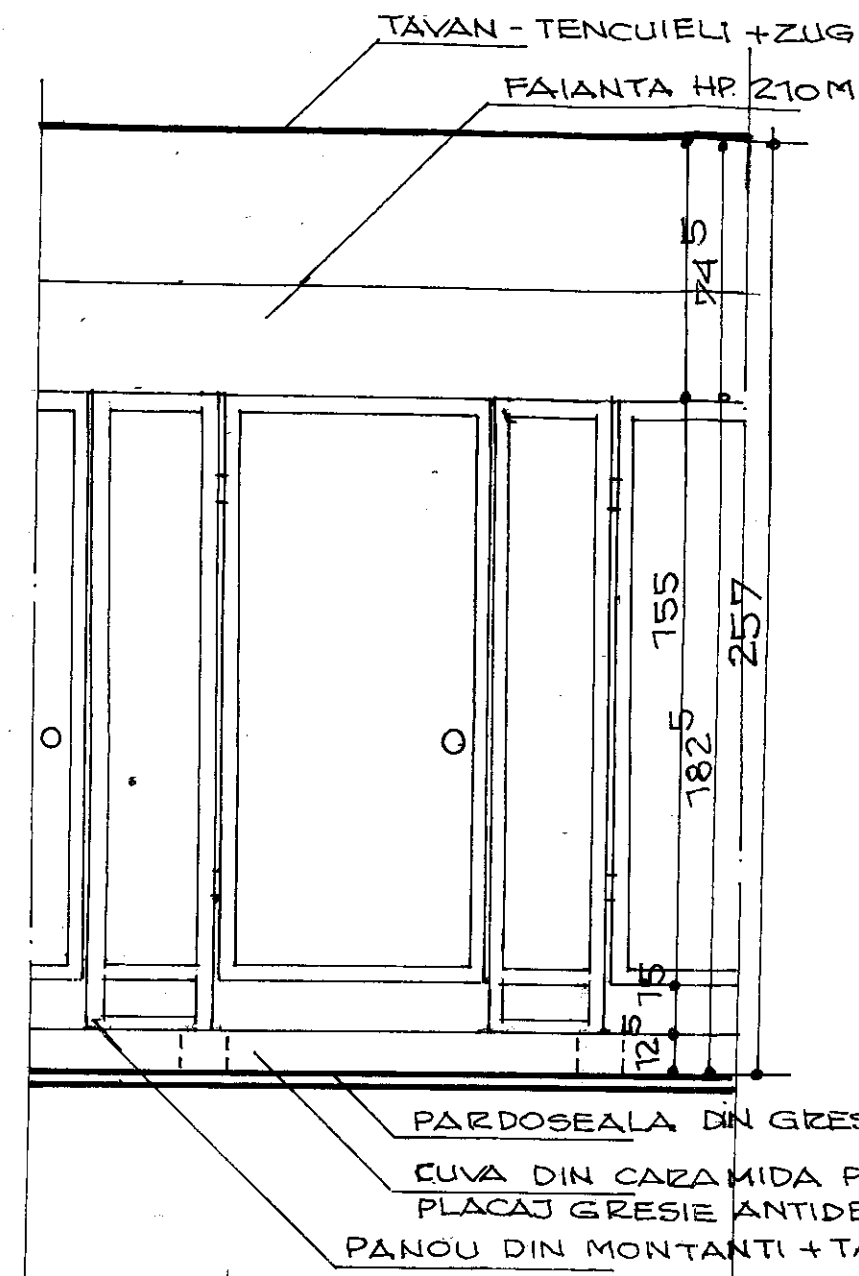
● VEDERE FRONTALA
