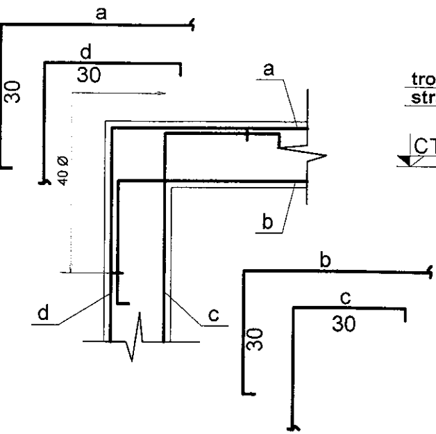
Detaliu rampa 3 - 3 SCARA 1:20
