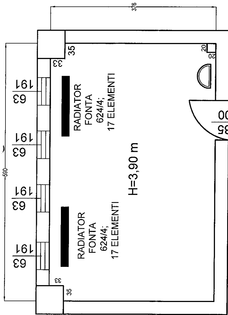
SCARA 1:50
